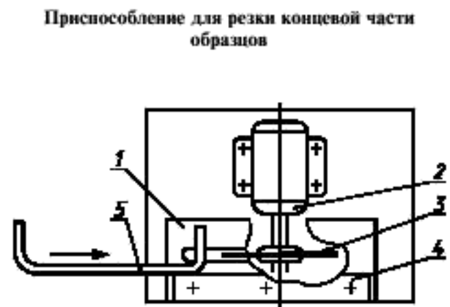
1 — стол; 2 — электродвигатель мощностью 300 Вт; 3 — отрезной диск на специальной бакелитовой основе (электроронд белый); 4 — упор; 5 — образец проволоки
